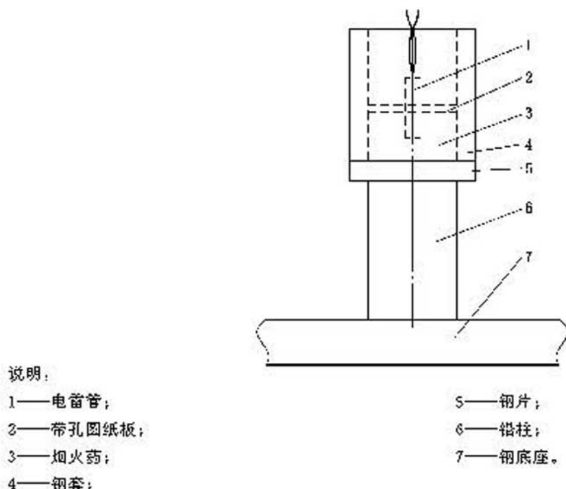
图 7 爆炸压缩铅柱装置示意图
