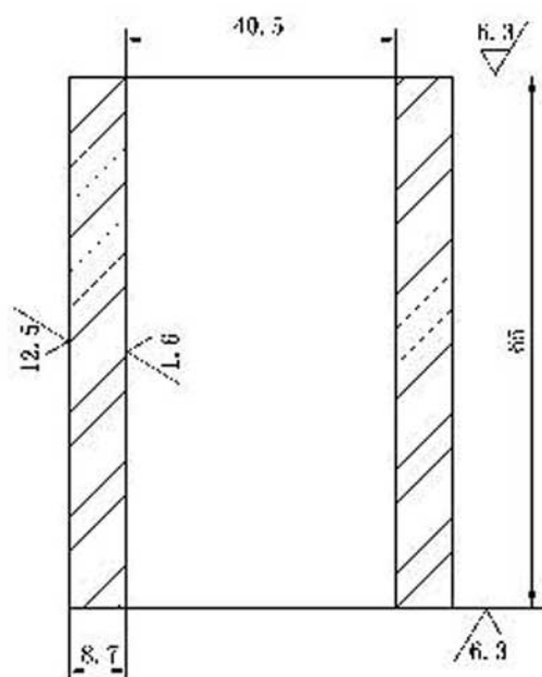
图 2 钢套
